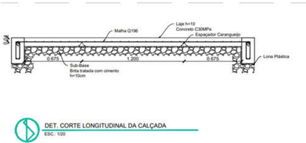
Figura 1 Recorte projeto estrutura do piso da calçada
