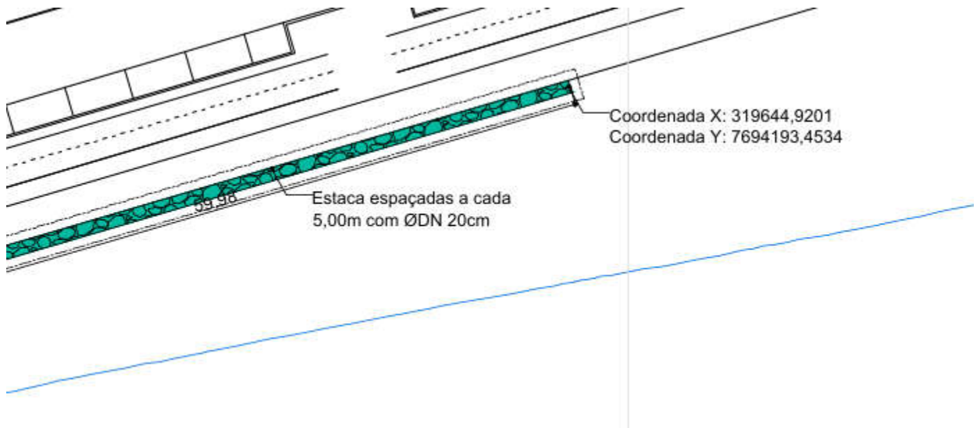
Figura 8 Recorte projeto de contenção
