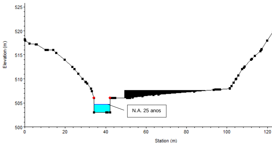
Figura 2-3: Perfil transversal da seção de escoamento no trecho em canal aberto do Córrego do Gordo para tempo de recorrência de 25 anos.
