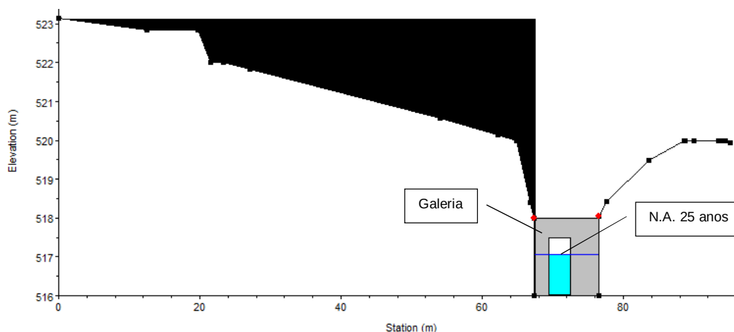
Figura 2-2: Perfil transversal da seção de escoamento no trecho em galeria do Córrego do Gordo para tempo de recorrência de 25 anos.
