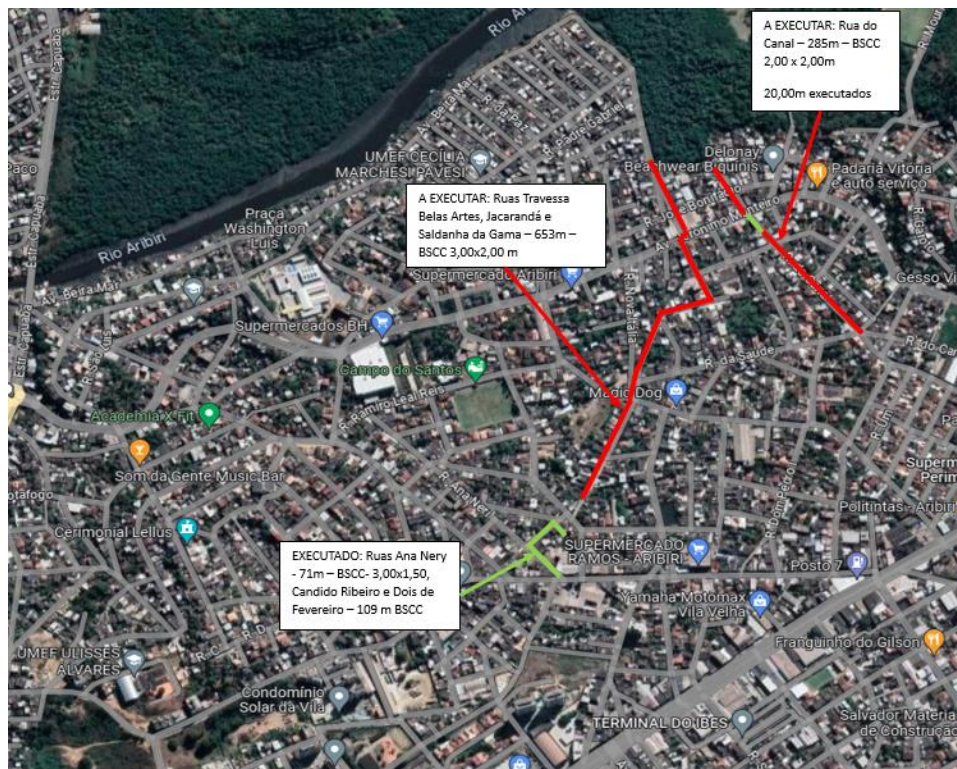
Figura 5 – Trechos de galerias pluviais a executar
