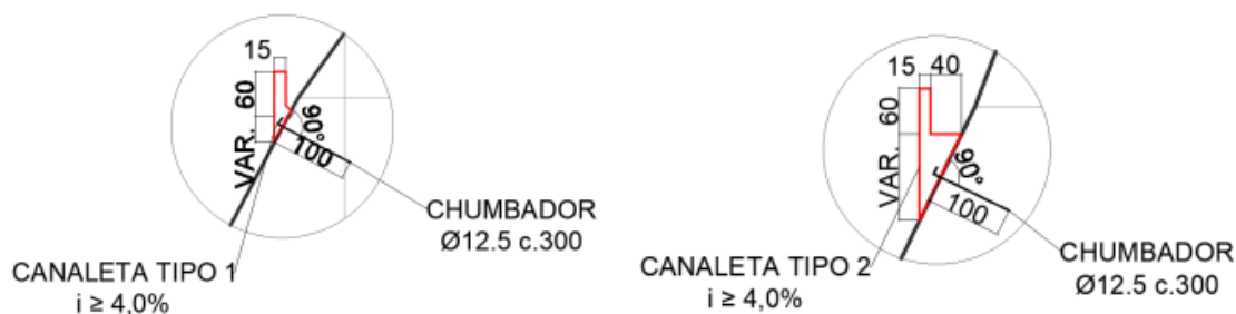
Figura 11 – Detalhes das Canaletas.
