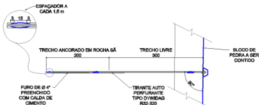
Figura 9 – Detalhes do Tirante.
